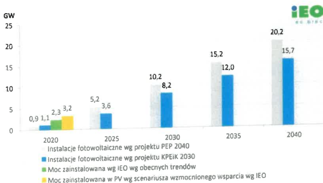
Rysunek 1 Prognoza rozwoju mocy fotowoltaicznych wg PEP 2040, KPEiK 2030 oraz scenariusz krótkoterminowy IEO na 2020. Oprac. IEO
